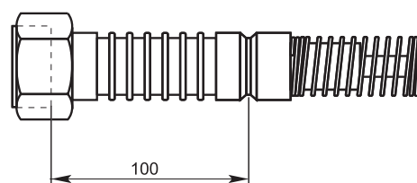
KS-5 waga 0,5 kg
