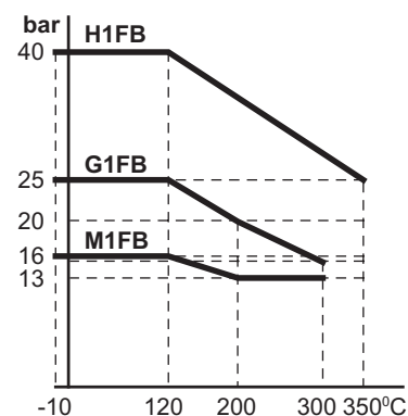
Wykres Temperatura - Ciśnienie DN 25-80
