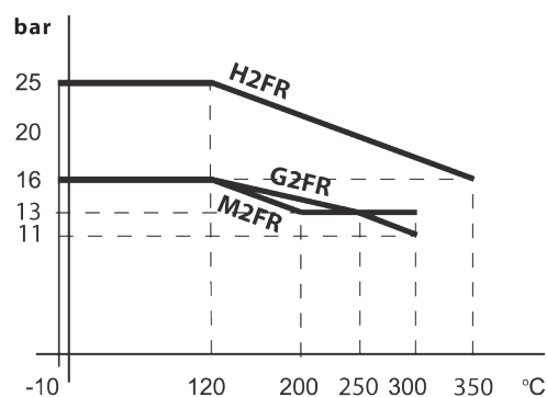
Wykres Temperatura - Ciśnienie DN 100-150
