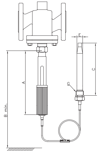
Wymiary zaworu
