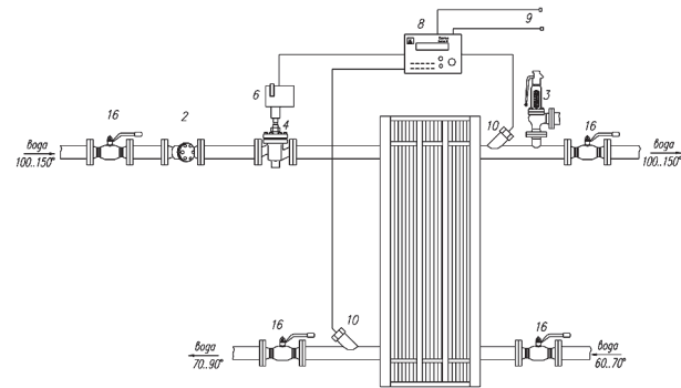
Schemat regulacji pogodowej
