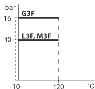
Wykres Temperatura - Ciśnienie DN 65-150
