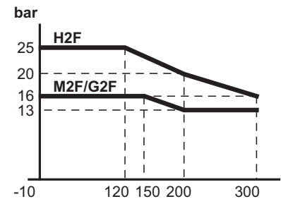
Wykres Temperatura - Ciśnienie
